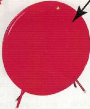
TIR120 โต๊ะกลมหน้าเหล็ก กว้าง 120 x สูง 75 ซม. เหล็กกลม 7/8 นิ้ว หน้า 0.7 มิล
