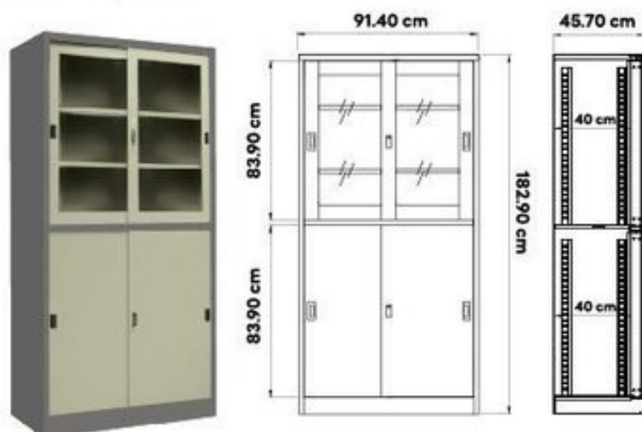
PK-301 ตู้เอกสารบานเลื่อน บนกระจก-ล่างทึบ
