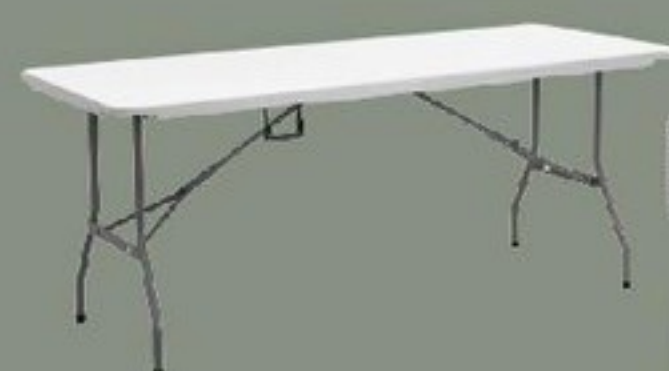
FP-181 โต๊ะพับอเนกประสงค์ 6 ฟุต แบบพับครึ่ง W 180 x D 75 x H 74 cm
