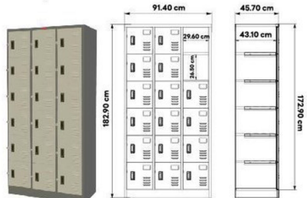
PK-018 ตู้ล็อกเกอร์ 18 ประตู
