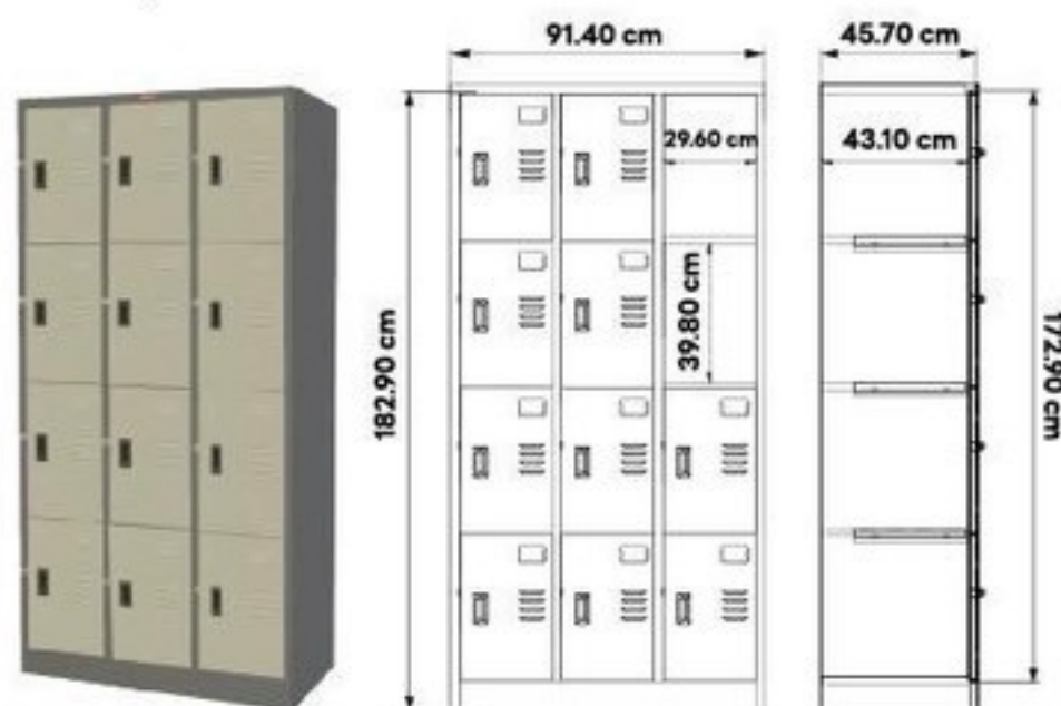
PK-012 ตู้ล็อกเกอร์ 12 ประตู
