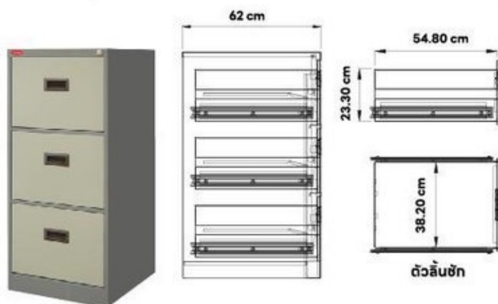
PC-103 ตู้เอกสาร 3 ลิ้นชัก ภายนอก W 46.1 x D 62 x H 101.6 cm ภายใน (ลิ้นชัก) W 38.2 x D 54.8 x H 23.3 cm PRICE 6,725.-
