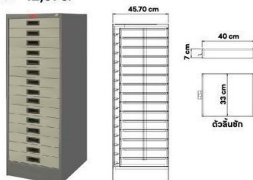
PC-215 ตู้เก็บแบบฟอร์ม 15 ลิ้นชัก
