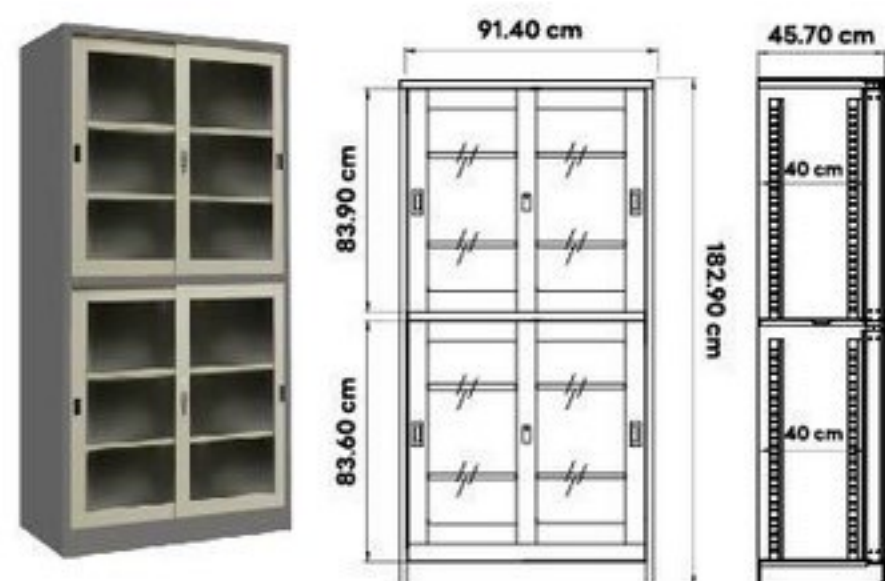
PK-302 ตู้เอกสารบานเลื่อน บนกระจก-ล่างกระจก
