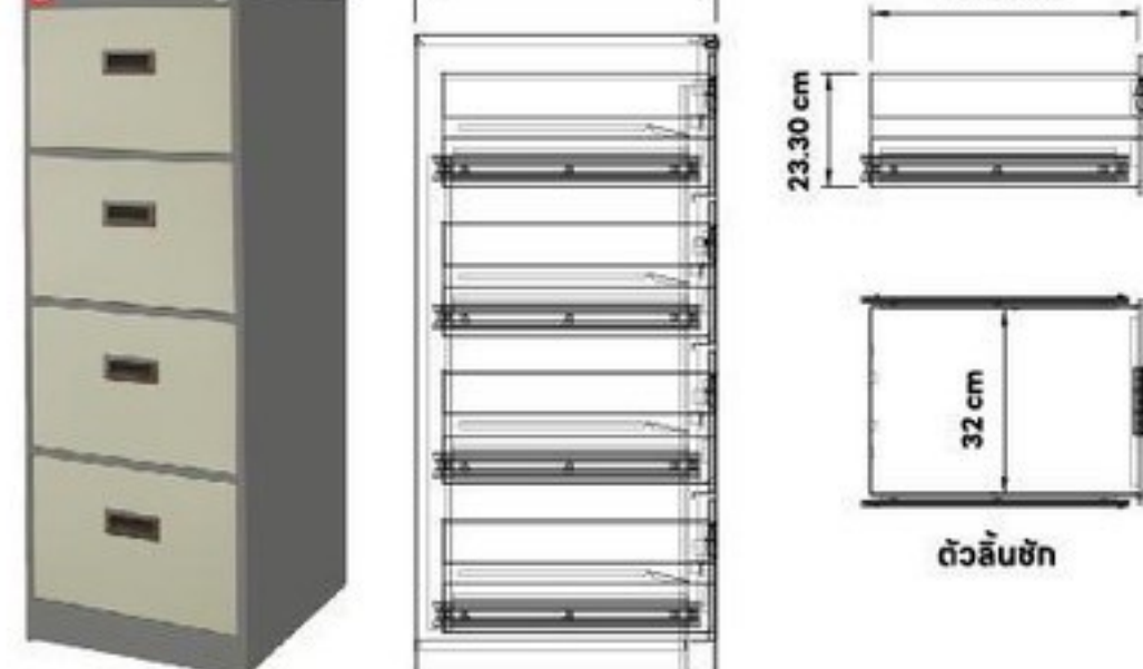
PC-104 ตู้เอกสาร 4 ลิ้นชัก ภายนอก W 46.1 x D 62 x H 132 cm ภายใน (ลิ้นชัก) W 32 x D 54.8 x H 23.3 cm PRICE 8,250.-
