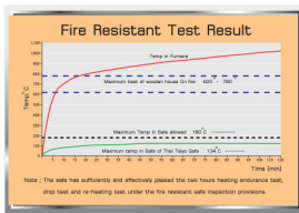
ภายใต้อุณหภูมิสูงถึง 1010°C Tested at temperature level 1010°C (1850°F)
